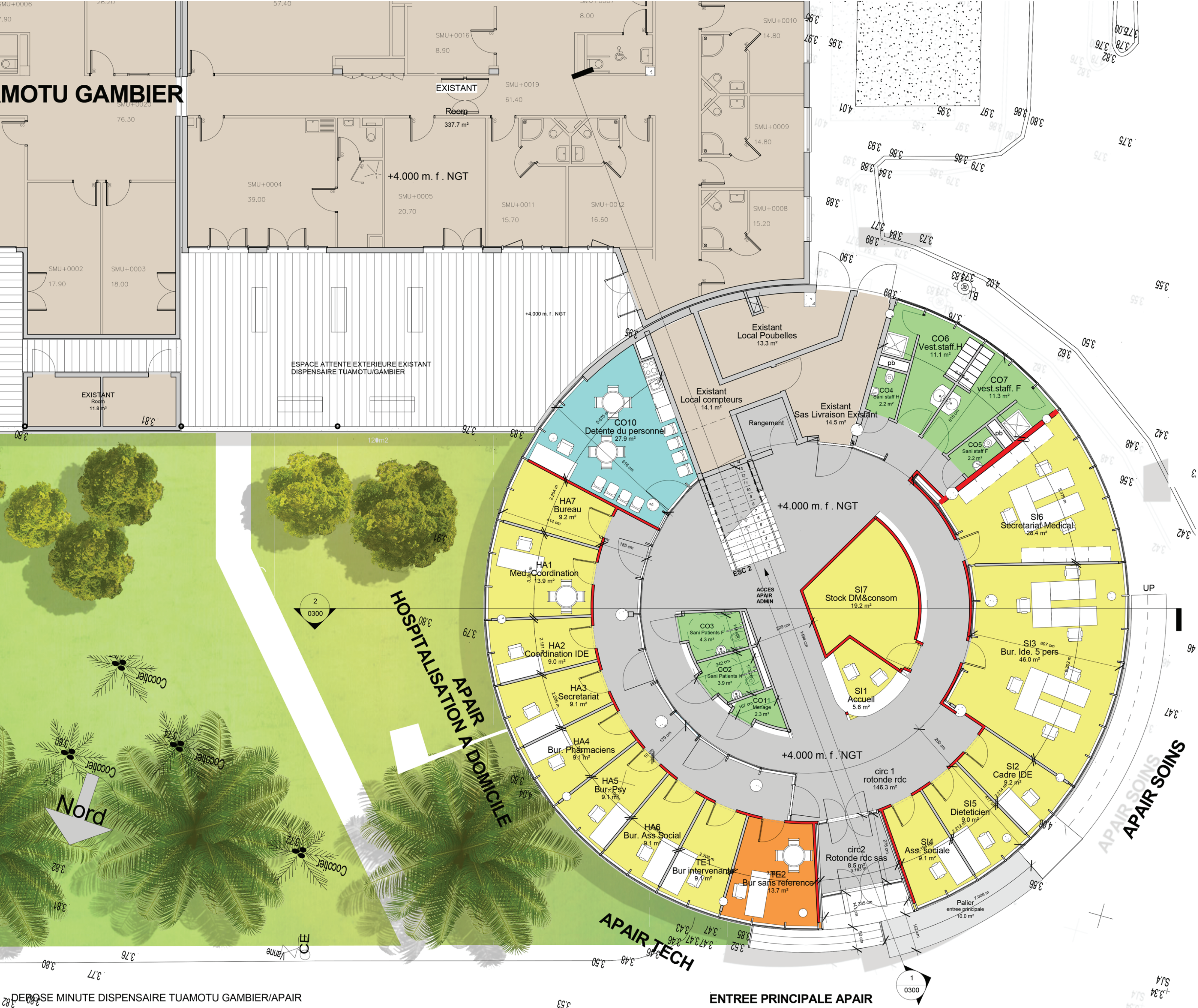
PLAN DU RDC ECH 1/100
