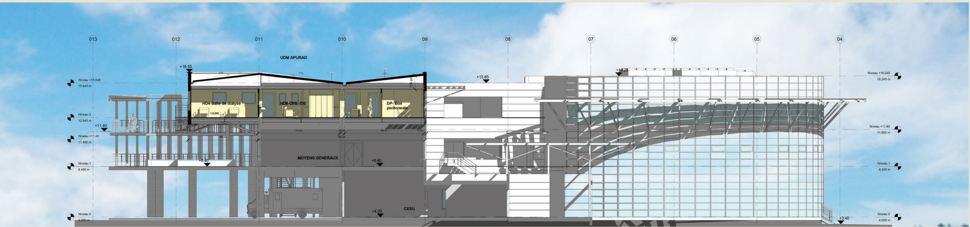
COUPE ECH 1/200
